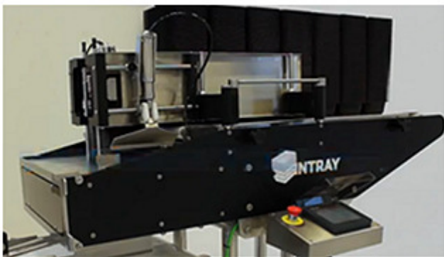
Intray bakkedispensermodul
